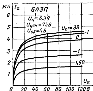
Анодные характеристики при U_{сз} = 4B .
