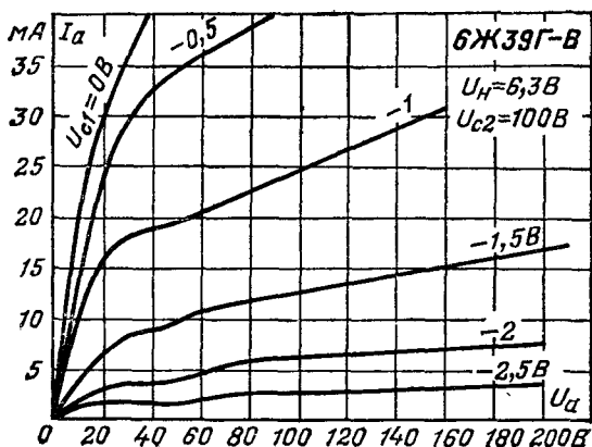
Анодные характеристики.
