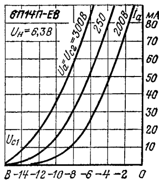
Анодно-сеточные характеристики.
