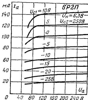
Анодные характеристики.
