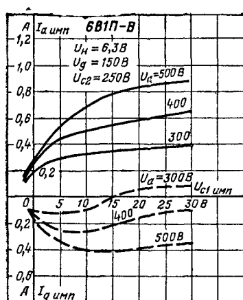
Импульсные (сплошные) и анодно-сеточные (пунктирные) и катодно сеточные характеристики.
