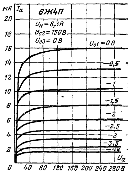
Анодные характеристики.
