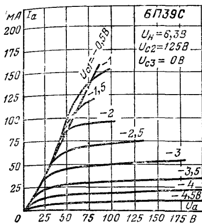
Анодные характеристики.
