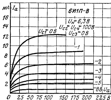
Анодные характеристики гектодной части.
