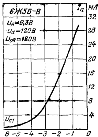
Анодно-сеточная характеристика.
