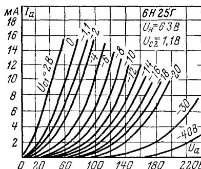
Анодные характеристики.
