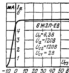
Анодно-сеточная характеристика по 3-й сетке.
