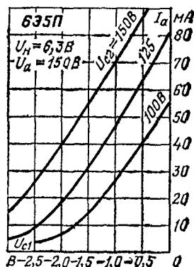
Анодно-сеточные характеристики.
