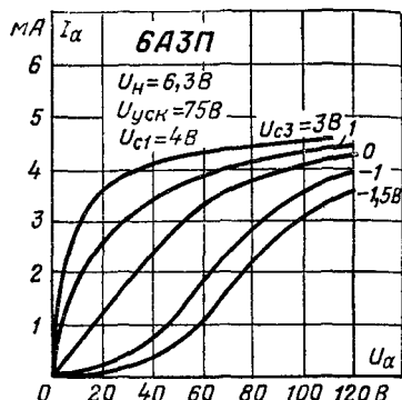
Анодные характеристики при U_{с1} = 4B .
