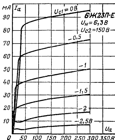
Анодные характеристики.
