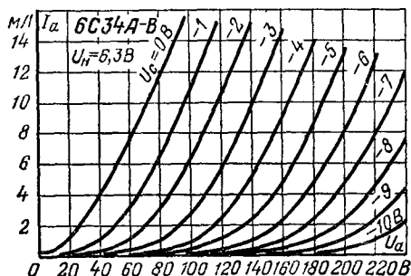
Анодные характеристики.
