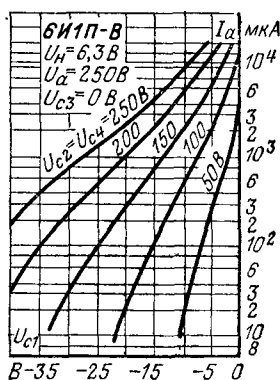
Анодно-сеточные характеристики гектодной части.
