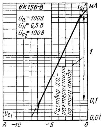
Анодно-сеточная характеристика.
