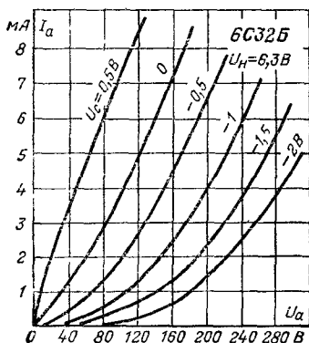
Анодные характеристики.
